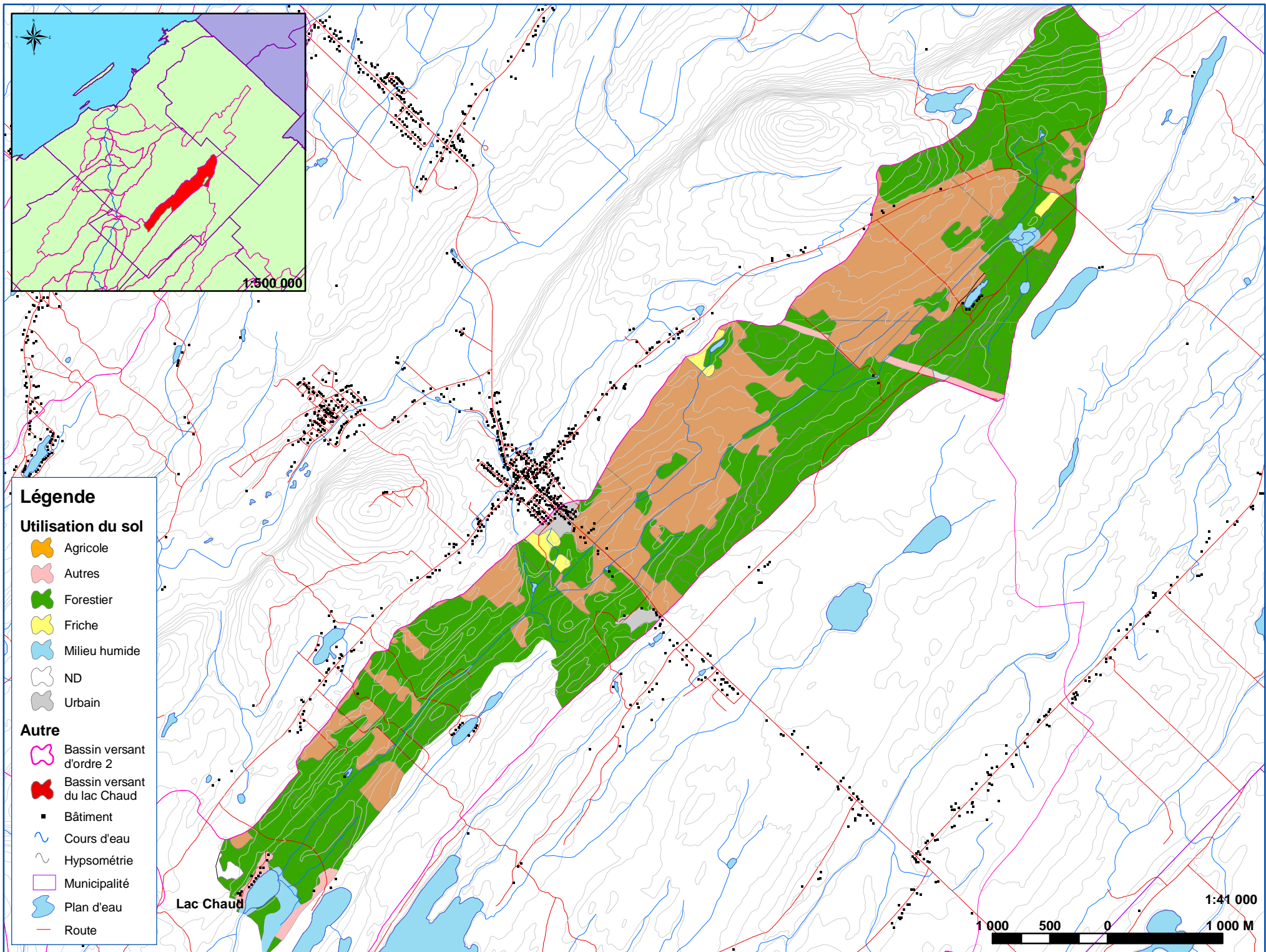
Figure 5.3.2 : Utilisation du sol du bassin versant du lac Chaud.
